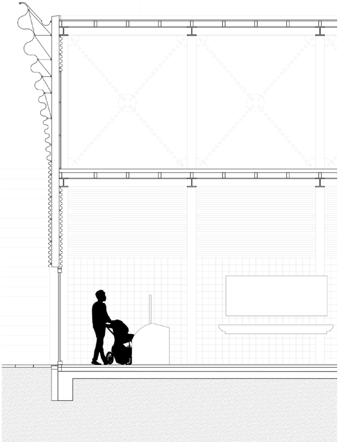
Section 1 : 50
